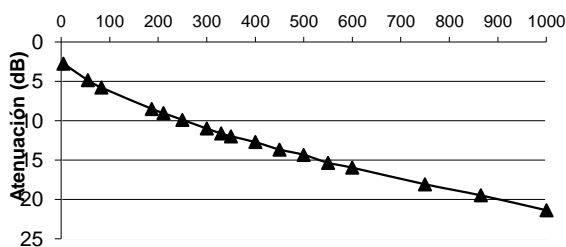
CURVA DE ATENUACIÓN DE SEÑAL Frecuencia (Mhz)
