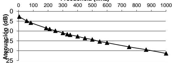
CURVA DE ATENUACIÓN DE SEÑAL Frecuencia (Mhz)
